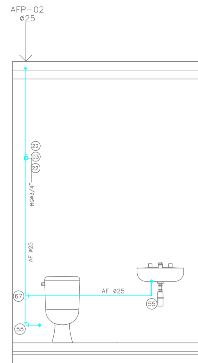
DIAGRAMA 02 - VISTA-01 INSTALAÇÕES LAVABO MASCULINO
