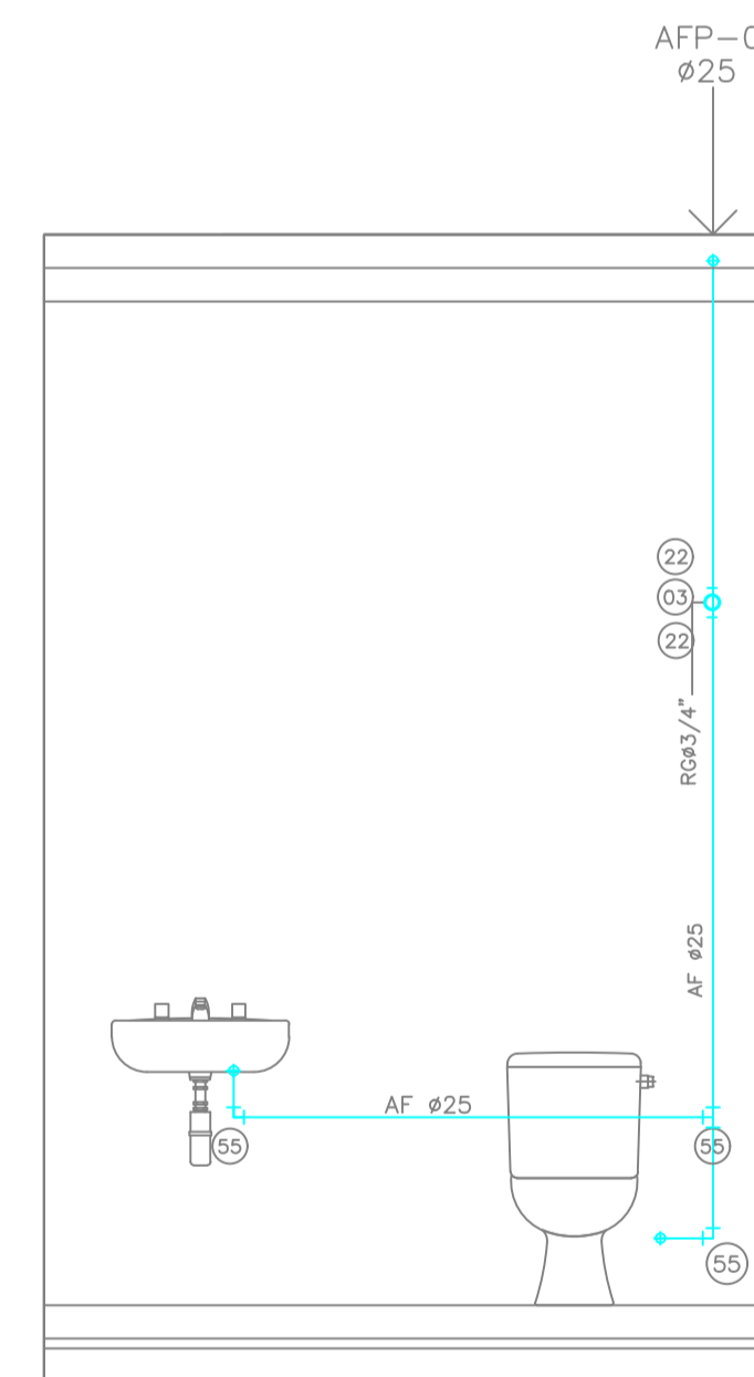
DIAGRAMA 01 - VISTA-01 INSTALAÇÕES LAVABO FEMININO
