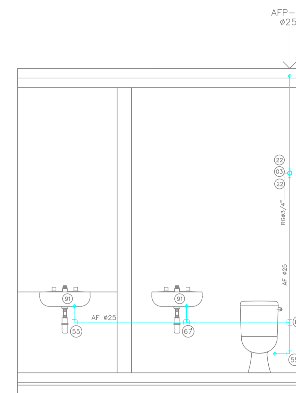
DIAGRAMA 04- VISTA-01 INSTALAÇÕES LAVABO - LAVATORIO
