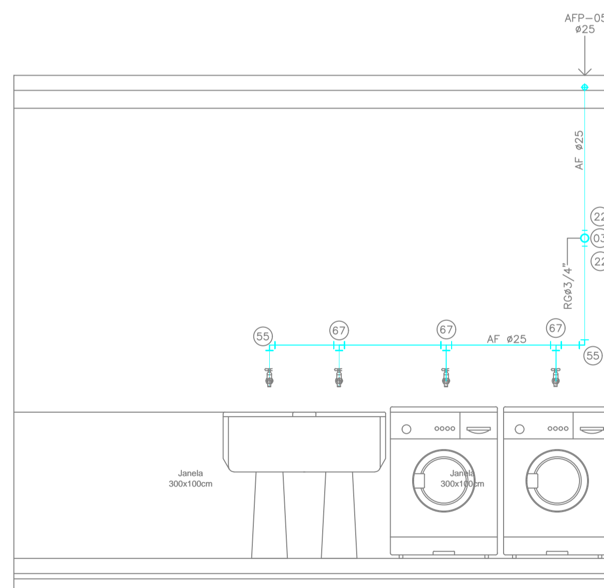
DIAGRAMA 05- VISTA-01 INSTALAÇÕES LAVANDERIA
