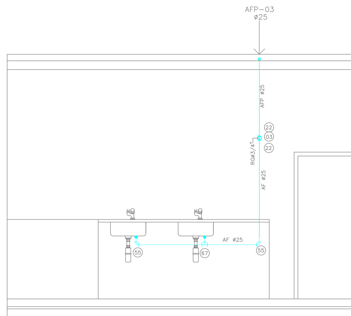
DIAGRAMA 03- VISTA-01 INSTALAÇÕES COZINHA
